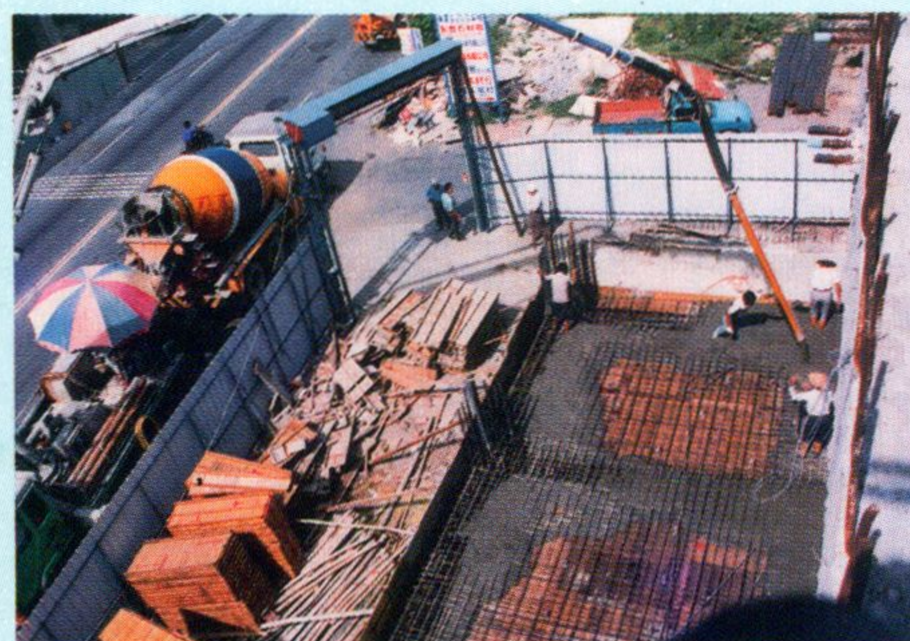
水泥車將攪拌已好的水泥砂，由泵浦高壓推上水泥而進行工作。
