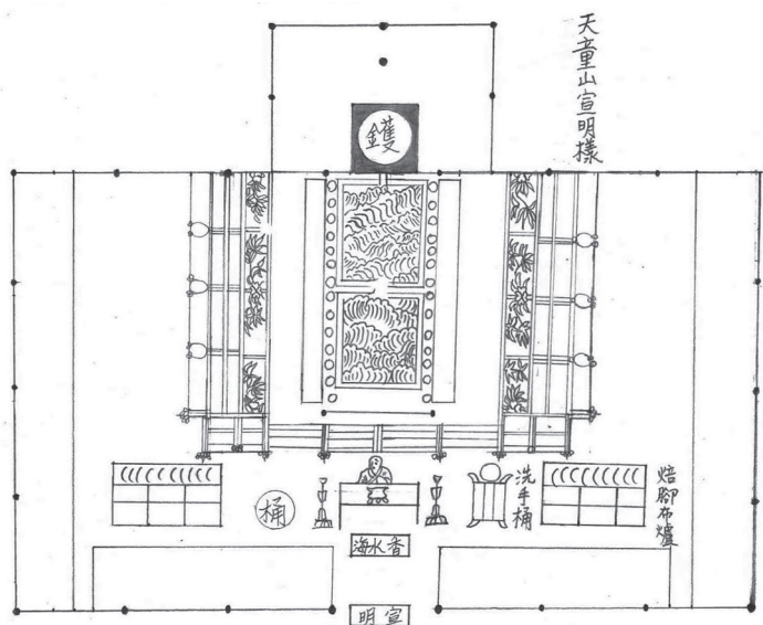
南宋天童寺的浴室內部設施（筆者手繪）
